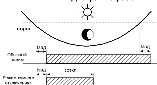
Диаграмма работы
