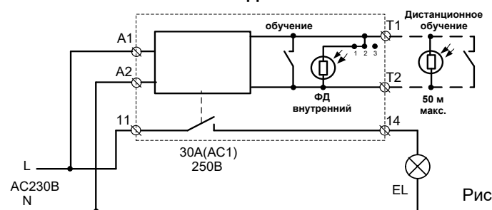
Схема подключения
